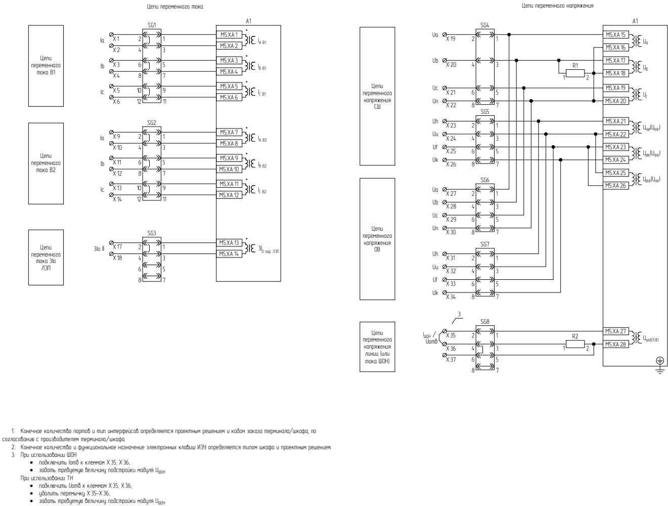
Рисунок Г.1 – Схема электрическая принципиальная (часть 1)
