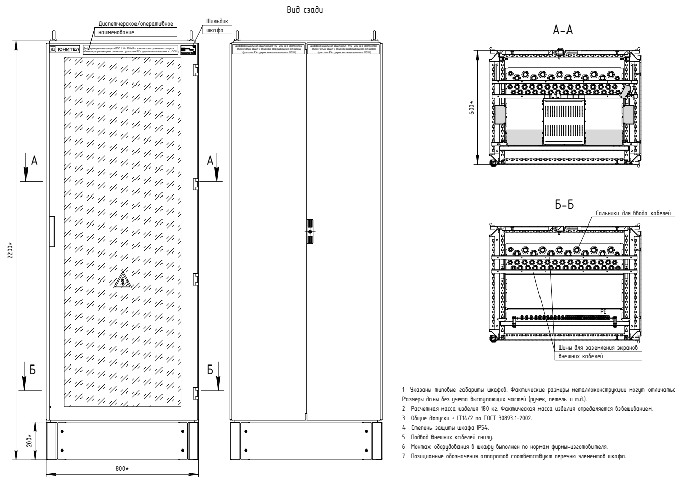
Рисунок В.1 – Чертеж общего вида (часть 1)
